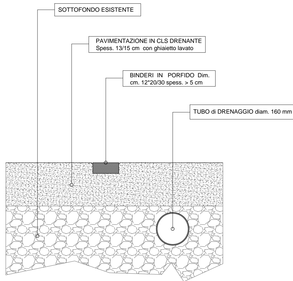
Particolare Pavimentazione
